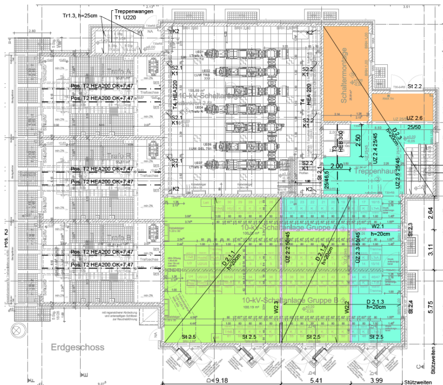
Positionsplan Decke über EG
